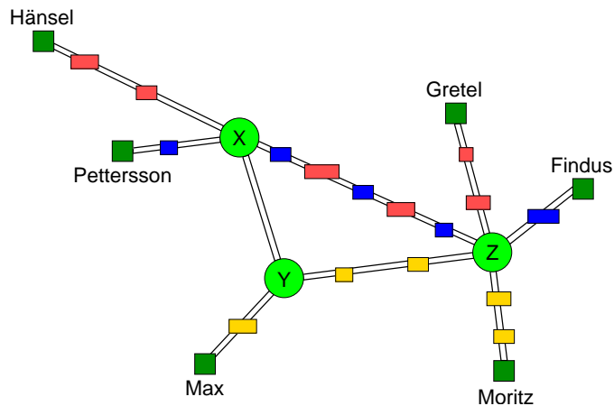
Abbildung 1.1-2.: Beispiel einer Paketvermittlung
